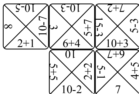
fig. 15 : dominos à deux dimensions
