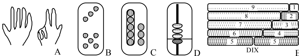
fig. 12 : Représentations des décompositions additives
