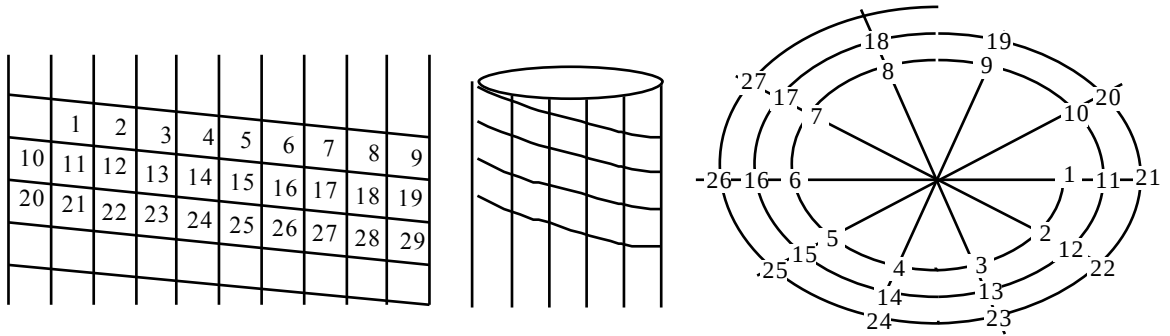
fig. 7 : dispositions en spirales
