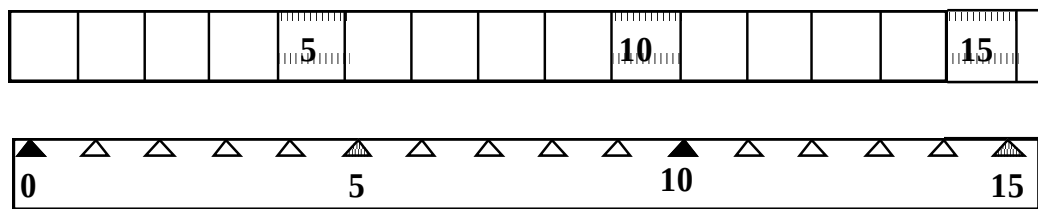
fig. 8 : graduation numérique
